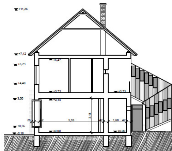
A-A metszet
