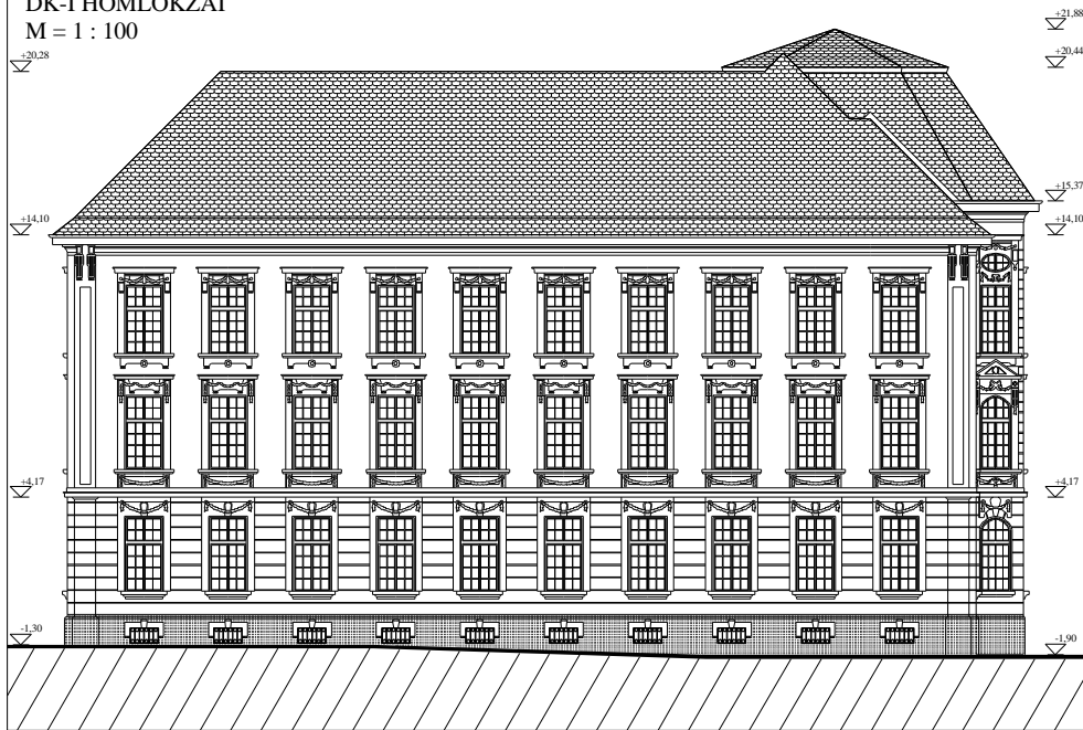
ÉNY-I HOMLOKZAT M = 1 : 100
