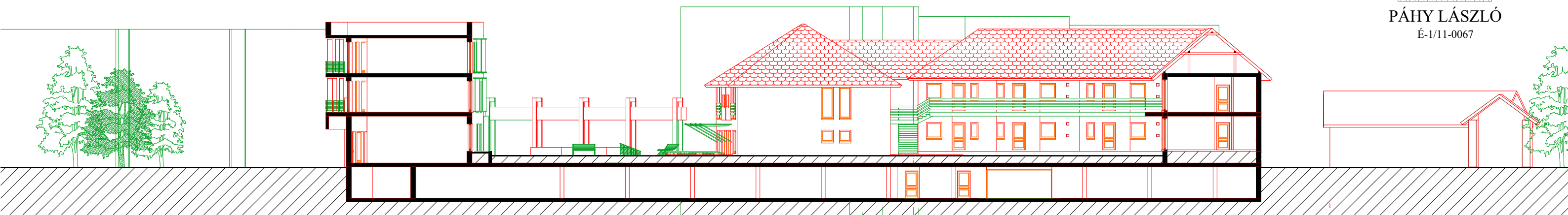
D-D METSZET M=1:200
