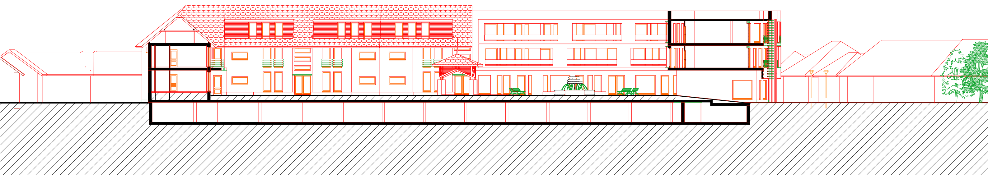
C-C METSZET M=1:200
