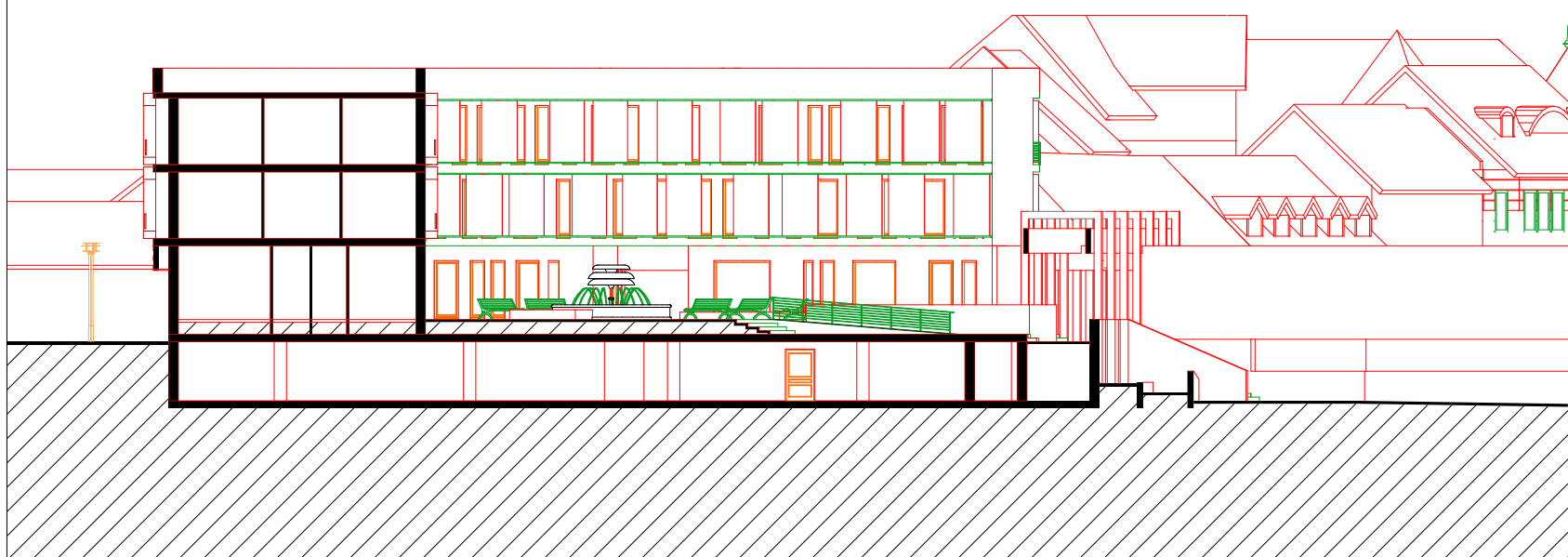
B-B METSZET M=1:200
