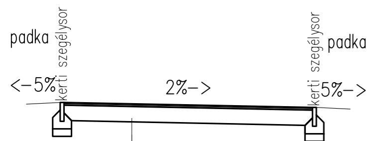
Egyesített gyalog- és kerékpárút
