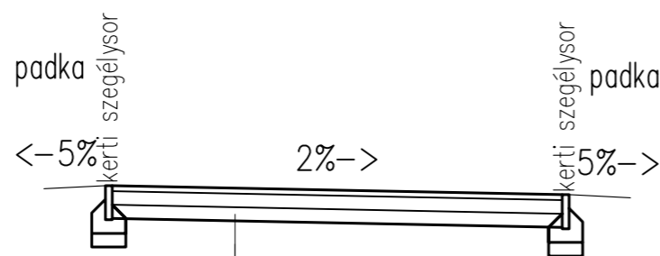
Egyesített gyalog- és kerékpárút
